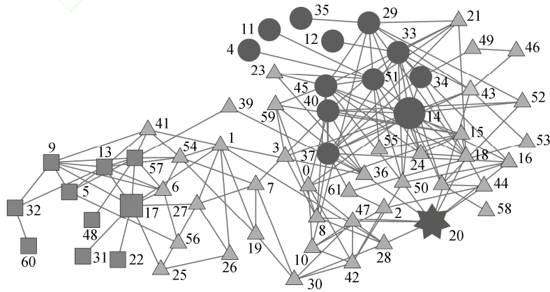
图 8 GS 算法在海豚社会网络上发现的社区
