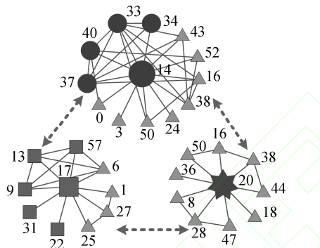
图 10 海豚社会网络上的 1 跳压缩
